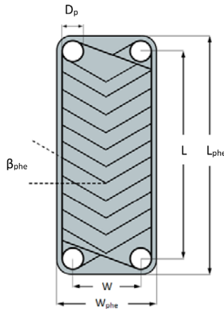
Fig. 4. PHE chevron plate.
