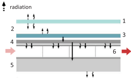
Fig. 10. PVT model.
